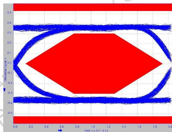
Eye Diagram (480Mbps)
