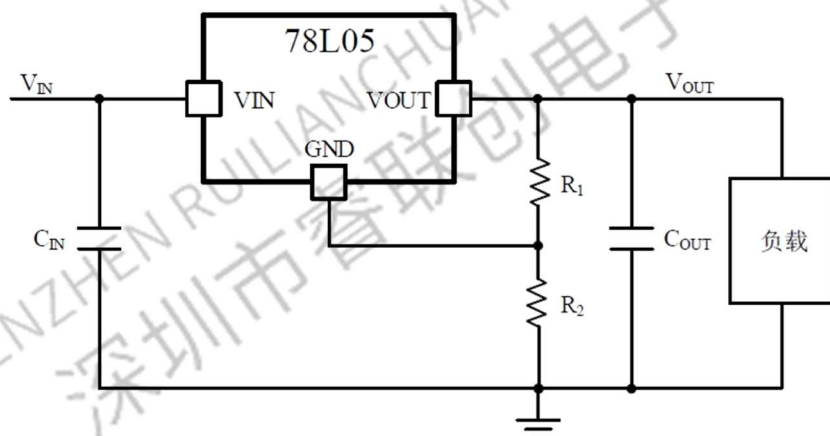
可调输出典型应用电路
